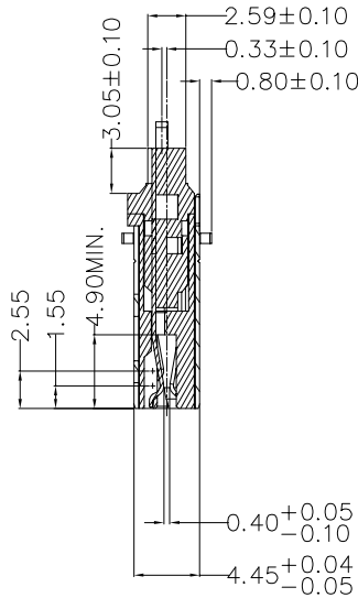
截面 A-A
